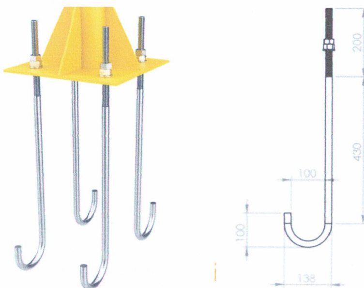
Figura 1 – Chumbadores metálicos tipo gancho
